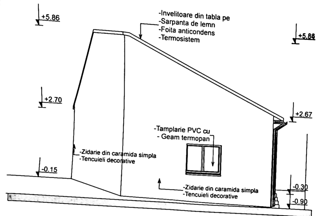
FATADA VEST SCARA 1:100
